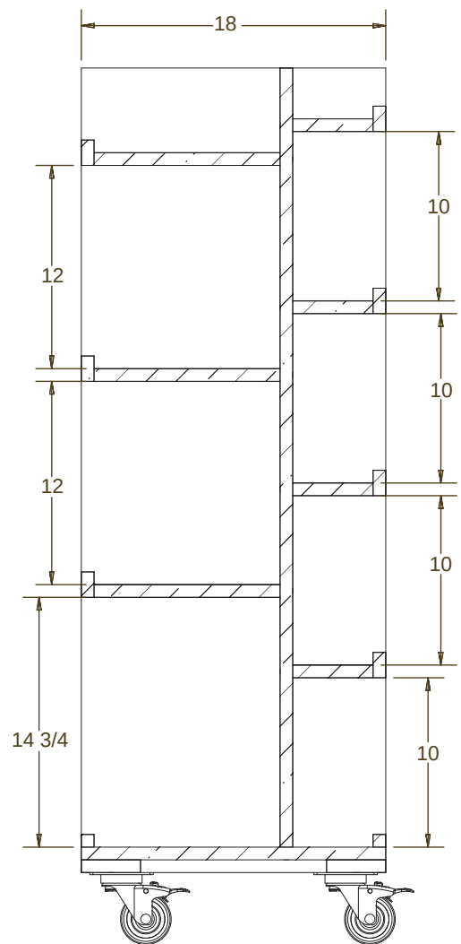
SECTION A-A
