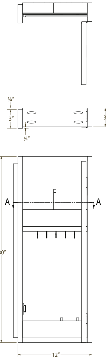
SECTION A-A
