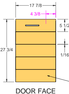
DOOR FACE
