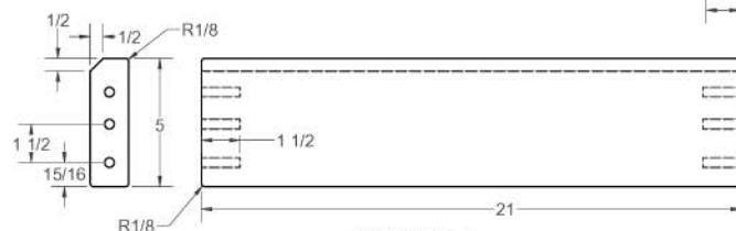
TOP RAILS - E
